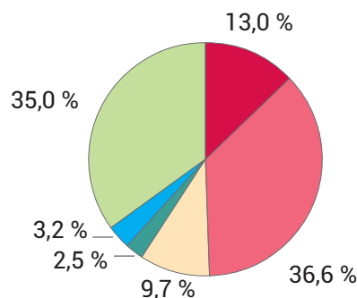
Energiemix Deutschland
